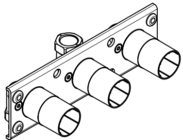
AXOR 800 45442180 / 45442187
