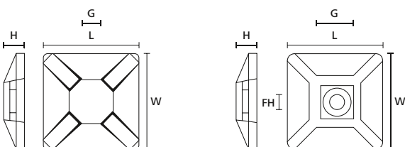
Zadel MB2A (zij- en bovenaanzicht)
