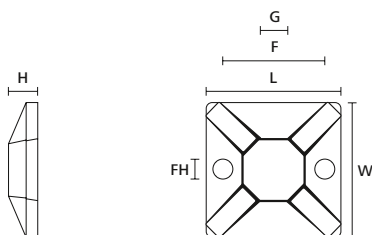
MB3-MB5 (zijaanzicht)
