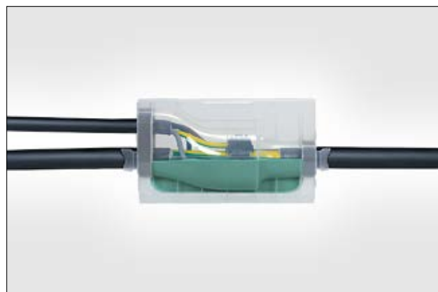
Parallele aftakmof PAH-4 140/420, huisaansluiting.
