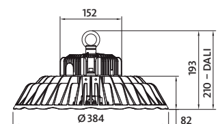
AURA CERTOS 120 W & 150 W
