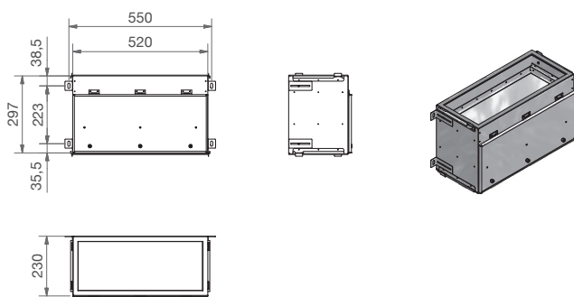
CW-P 520 - Aansluitplaat DN160
