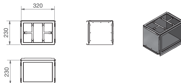
CW-M 320 - Verdeelplaat 6XDN90/P - RLC
