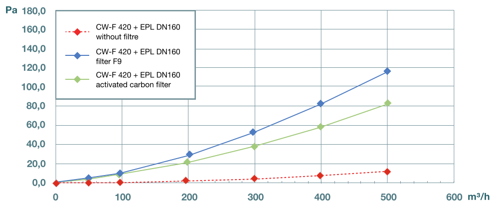
Drukverlies - CW-F 420 (enkel/in serie) + CW-P 420 DN160
