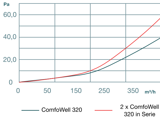
Drukverlies - CW-S 320 (enkel/in serie) + CW-P 320 DN160
