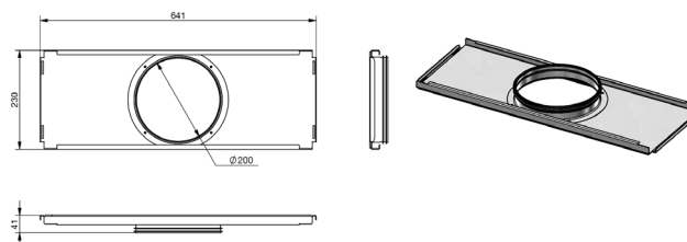
CW-P 625 - Aansluitplaat DN200
