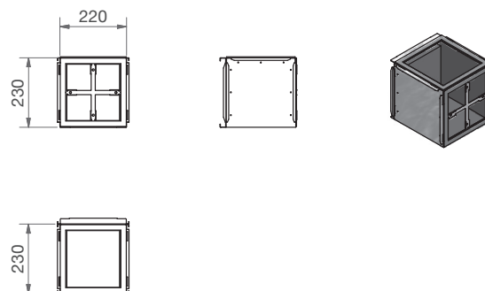
CW-M 220 - Verdeelplaat 4XDN90/P - RLC
