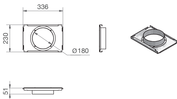
CW-P 320 - Aansluitplaat DN180
