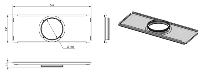
CW-P 625 - Aansluitplaat DN180
