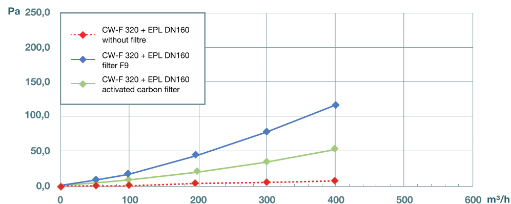
Drukverlies - CW-F 320 (enkel/in serie) + CW-P 320 DN160
