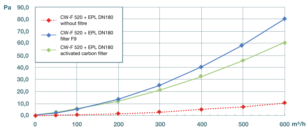
Drukverlies - CW-F 520 (enkel/in serie) + CW-P 520 DN180
