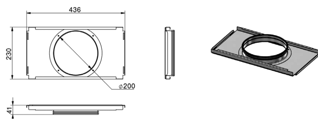
CW-P 420 - Eindplaat DN200
