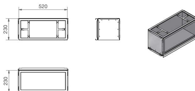
CW-M 520 - Verdeelplaat 10XDN90/P - RLC
