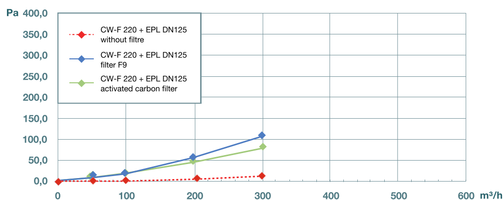
Drukverlies - CW-F 220 (enkel/in serie) + CW-P 220 DN125
