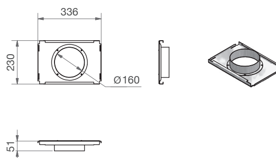
CW-P 320 - Aansluitplaat DN160
