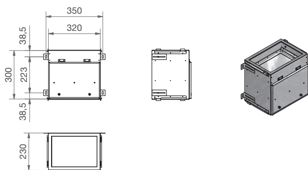
CW-P 320 - Aansluitplaat DN125
