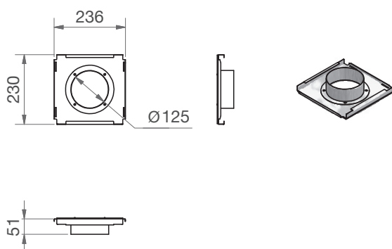
CW-P 220 - Eindplaat DN125
