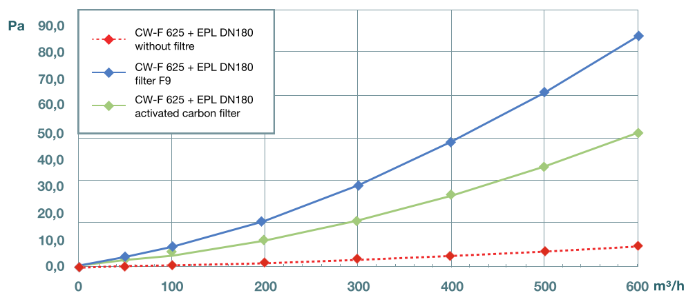
Drukverlies - CW-F 625 (enkel/in serie) + CW-P 625 DN180
