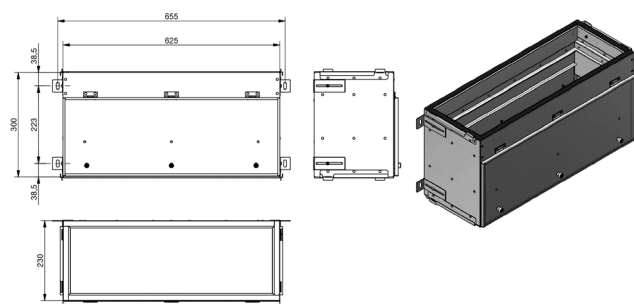
CW-P 625 - Aansluitplaat DN180
