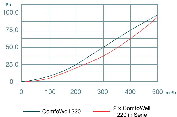
Drukverlies - CW-S 220 (enkel/in serie) + CW-P 220 DN125
