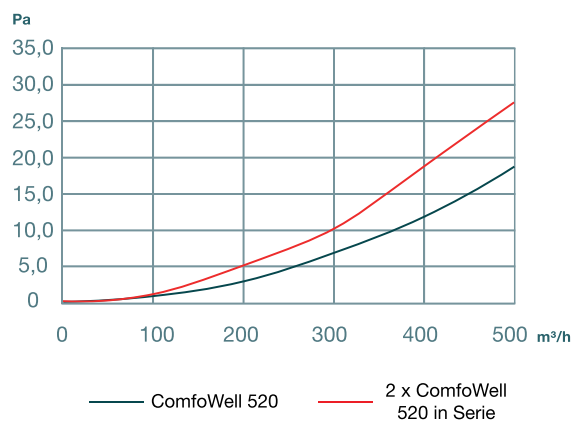
Drukverlies - CW-S 520 (enkel/in serie) + CW-P 520 DN180
