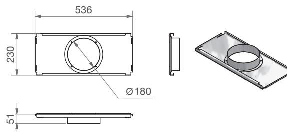
CW-P 520 - Aansluitplaat DN180
