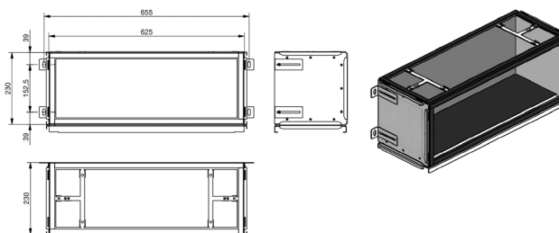
CW-M 625 - Verdeelplaat 12XDN90/P - RLC
