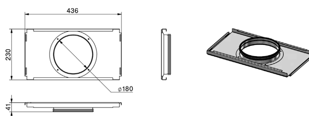
CW-P 420 - Eindplaat DN180
