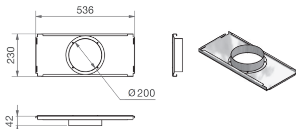
CW-P 520 - Aansluitplaat DN200
