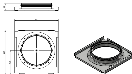
CW-K 220 - Aansluitplaat CA Flex 250/350 DN160 (excentrisch)
